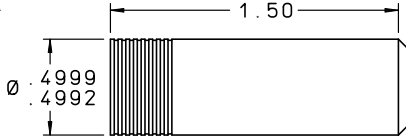
INSERT
