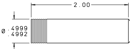
INSERT
