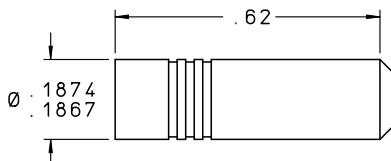
INSERT
