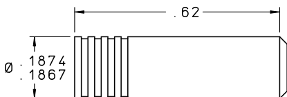
INSERT
