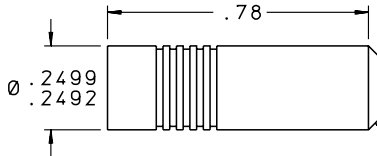
INSERT
